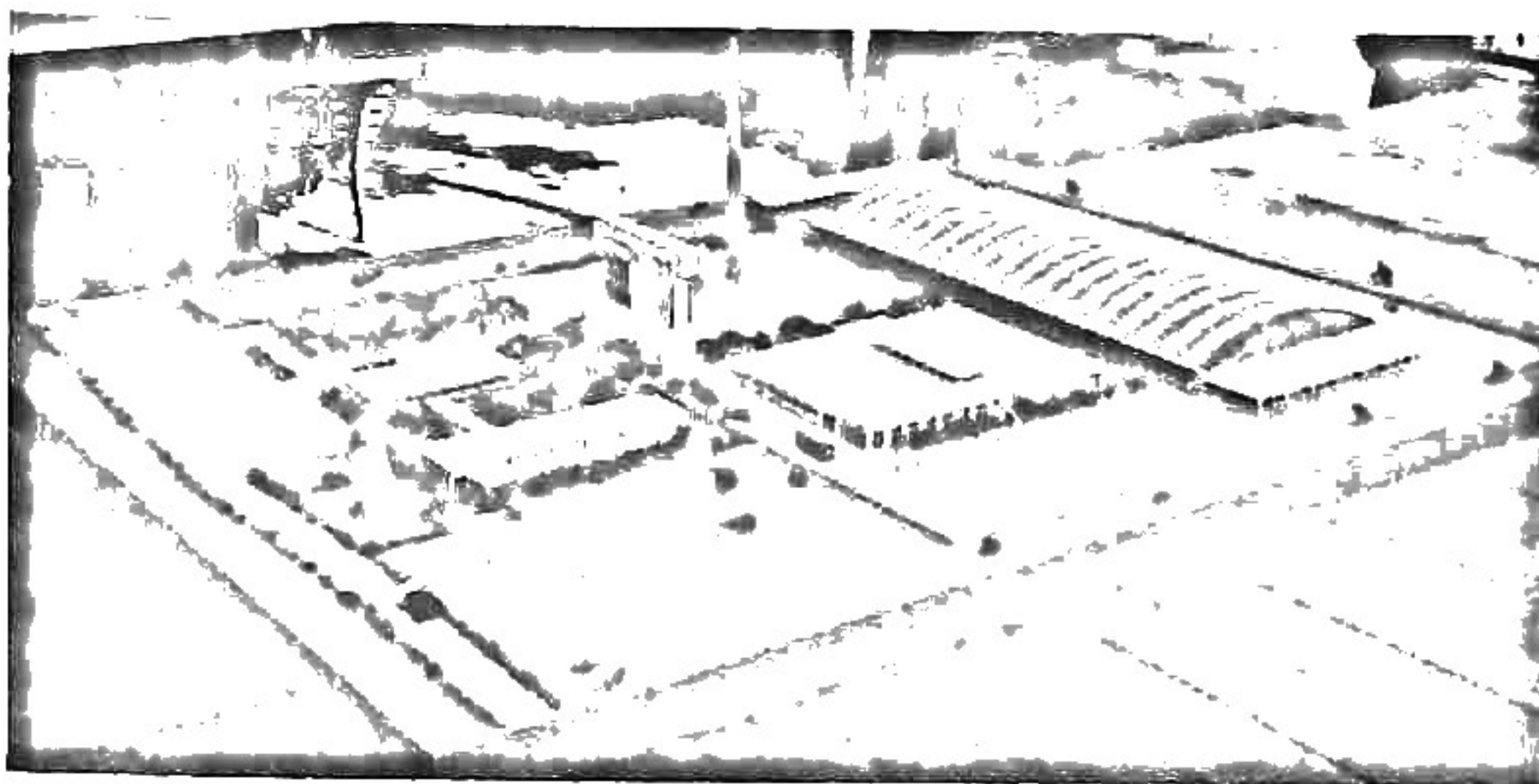
Plastico del progetto d'impianto industriale della Azienda Municipalizzata per la Nettezza Urbana, comprendente: Centrale di incenerimento dei rifiuti solidi urbani; Autorimessa - officina - magazzino - servizi per il personale; Impianto centrale per lavanderie. Il plastico è stato esposto alla Fiera di Bologna.
